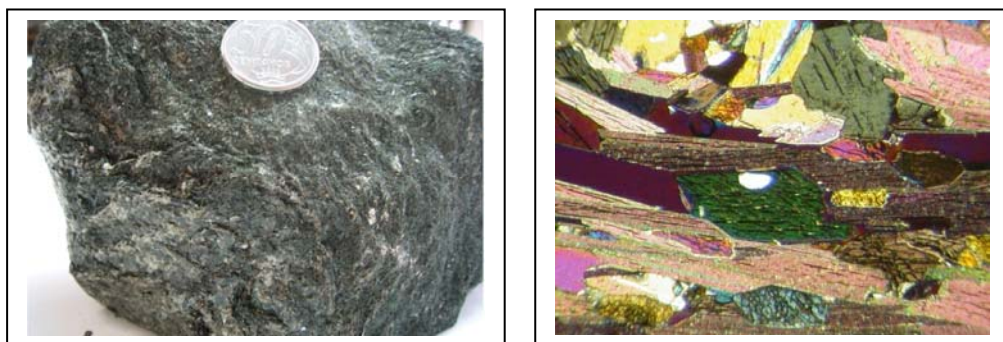
Figura 2 – (2A) Biotita-flogopita xisto, rocha hospedeira da esmeralda dos depósitos do distrito de Nova Era-Itabira, Minas Gerais. (2B) Fotomicrografia do biotita- flogopita xisto destacando lamelas de biotita e flogopita em associação com anfibólio da matriz meta-ultrabásica reliquiar.
