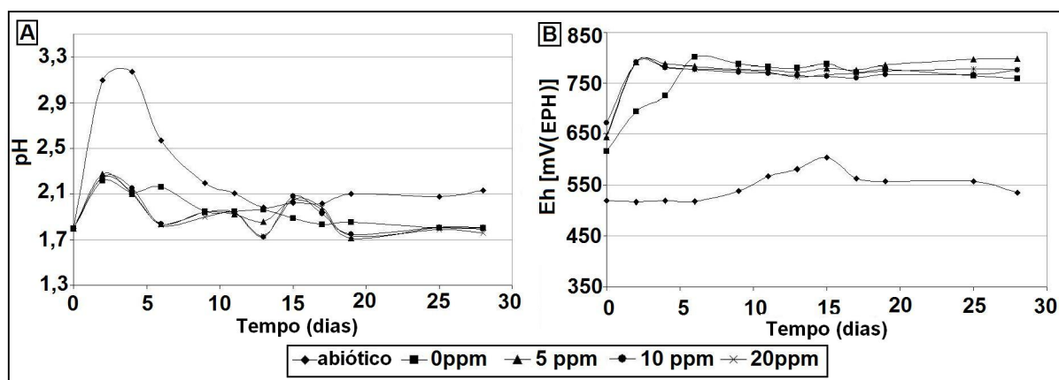
Figura 1. Variação de pH (A) e Potencial de oxi-redução (B) nos experimentos de biolixiviação em frascos agitados.
