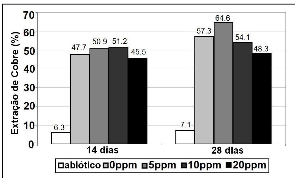
Figura 2. Extração de cobre nos experimentos de biolixiviação.
